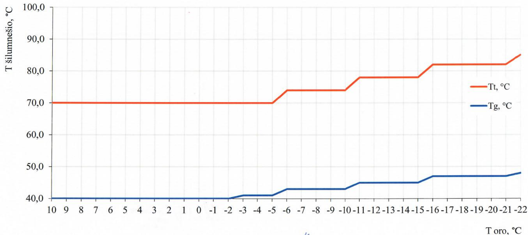
Temperatūrinis grafikas pagal 85-70 °C Skaičiuotina patalpų temperatūra 18 °C
